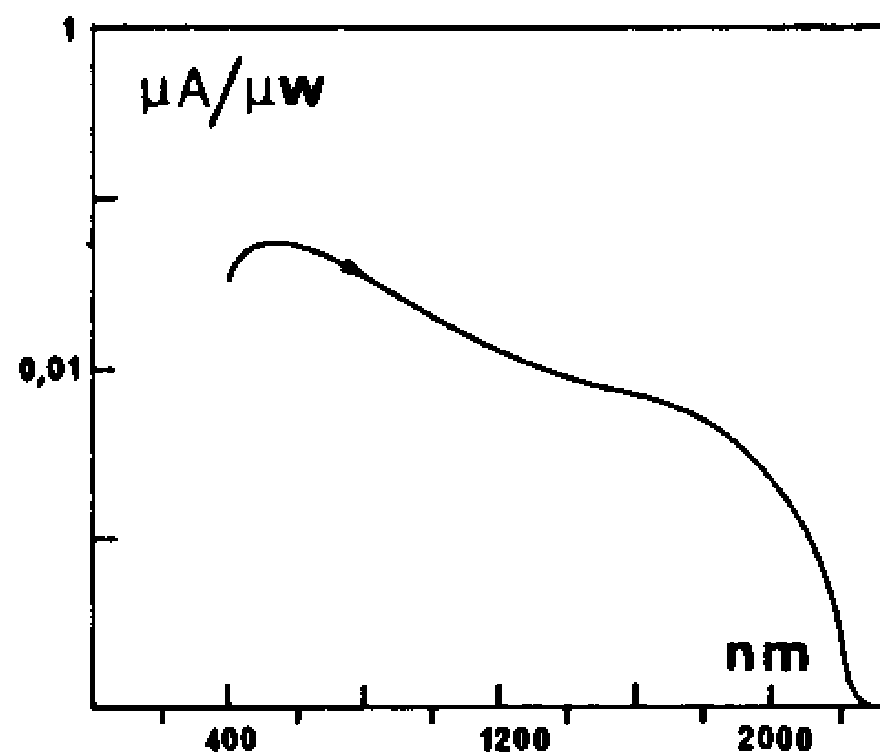
Σχ. 1: Φασματική απόκριση του σωλήνα N214-02 της HAMAMATSU
